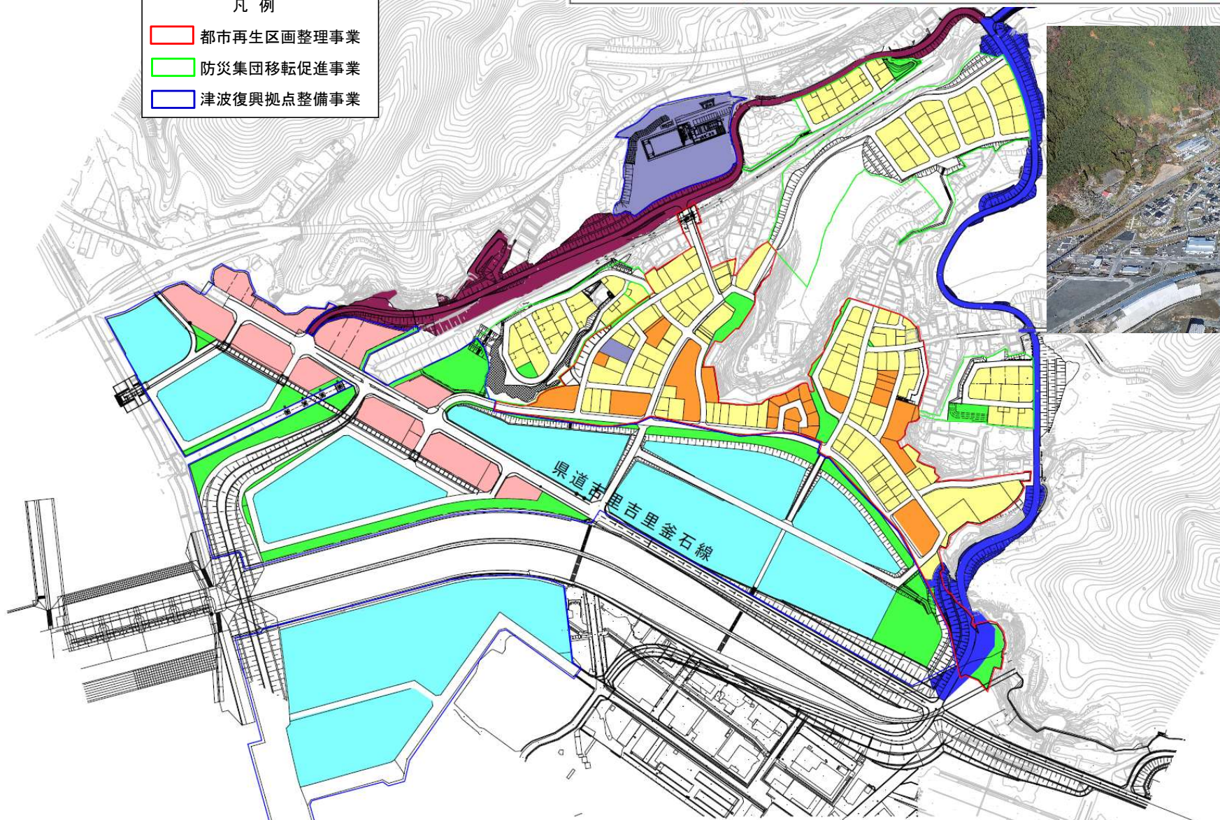
安渡地区全体計画平面図
