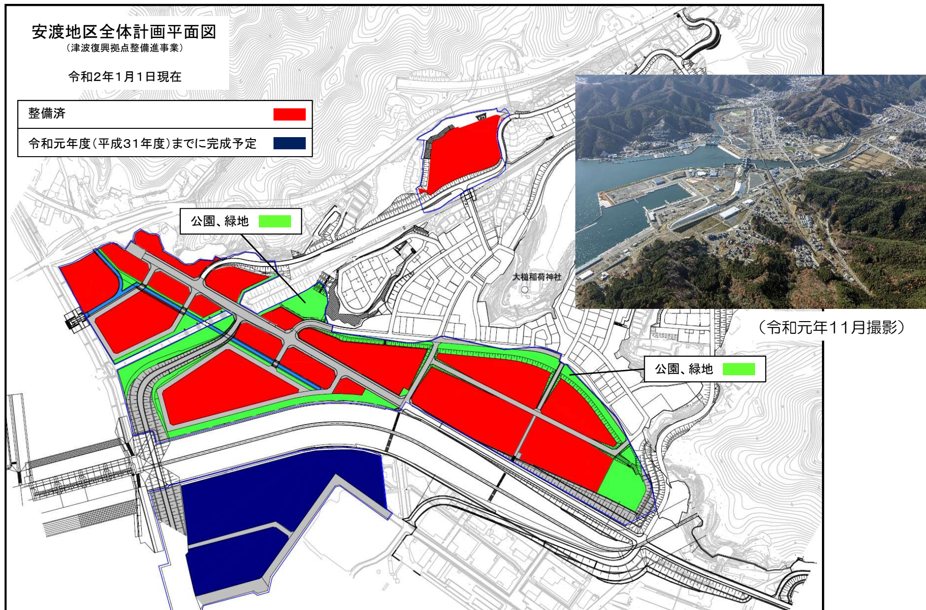
安渡地区津波復興拠点事業(19.9ha)
