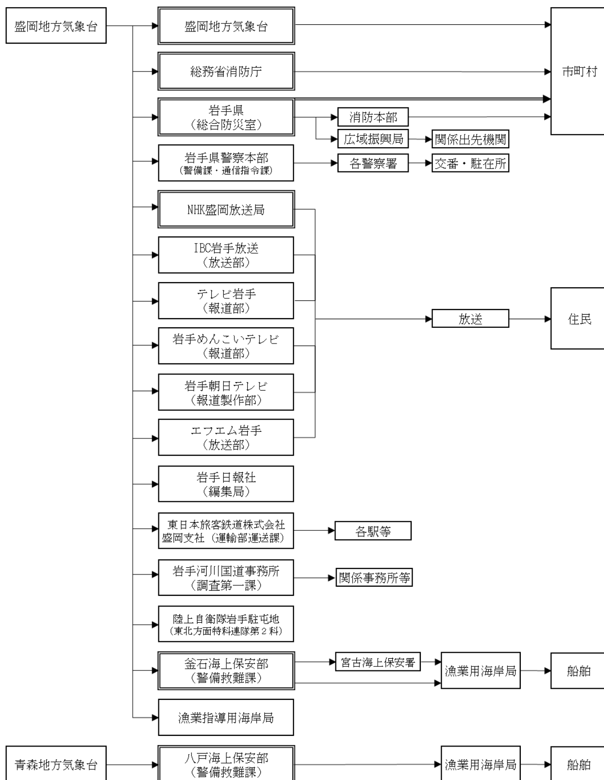
別図 1 (気象警報等伝達系統図)
