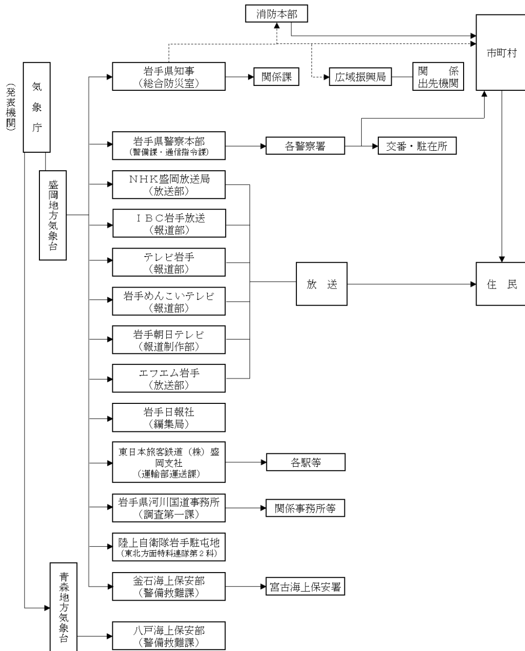
別図4（地震及び津波に関する情報伝達系統図）
